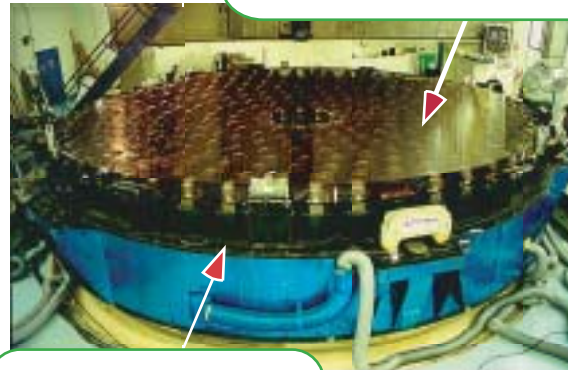
アクチュエータ： 鏡をささえる261本のロボットアーム
